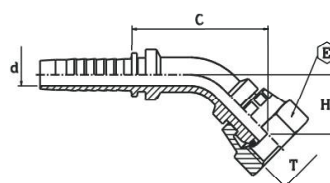
BSP FEMALE 60° FLARE 45° ELBOW WITH O'RING CRIMPED NUT FEMMINA 45° BSP SV. 60° CON O'RING DADO PINZATO 030145
