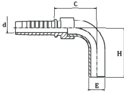
METRIC STAND PIPE 90° ELBOW - WELDED FEMMINA 90° TUBOLARE SALDATA 30364
