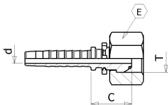
BSP FEMALE 60° FLARE WITH O'RING FEMMINA BSP SV. 60° CON O'RING 030121
