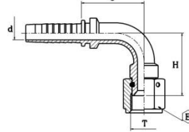
JIC FEMALE 37° FLARE 90° ELBOW WITH THRUST WIRE NUT FEMMINA 90° JIC SV. 37° CONDADO SPINATO 03 0262
