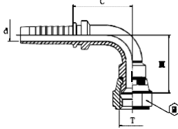
JIC FEMALE 37° FLARE 90° ELBOW FEMMINA 90° JIC SV. 37° 0 30260
