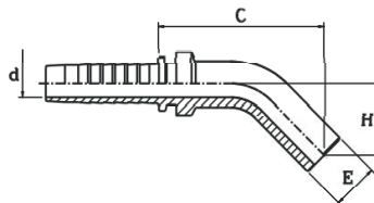
FEMMINA 45° TUBOLARE PEZZO UNICO (030343)
