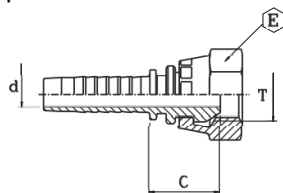
BSP FEMALE 60° FLARE FEMMINA BSP SV. 60° pinzato 030120
