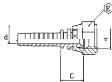
JIC FEMALE 37°FLARE FEMMINA JIC SV 37° 030220
