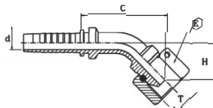
FEMMINA 45° BSP SV. 60° 030143 dado spinato
