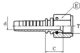
JICFEMALE37°FLAREWITHTHRUSTWIRENUT FEMMINAJICSV.37°CON DADO SPINATO 030223
