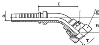
FEMMINA 45° BSP SV. 60° 030140 dado pinzato
