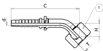
BSP FEMALE 60° FLARE 45° ELBOW WITH O'RING FEMMINA 45° BSP SV. 60° CON O'RING 030141
