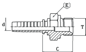
BSP PARALLELMALE 60° FLARE
