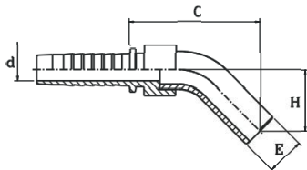
FEMMINA 45° TUBOLARE SALDATA (030342)
