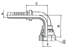
FEMMINA 90° BSP SV. 60° 30160
