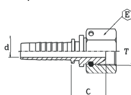
BSP FEMALE 60° FLARE WITH O-RING FEMMINA BSP SV. 60° CON O-RING spinato 030122
