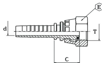
BSP FEMALE 60° FLARE WITH O'RING CRIMPED NUT FEMMINA BSP SV. 60° CON O'RING PINZATO 030122
