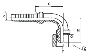
FEMMINA 90° BSP SV. 60° CON DADO SPINATO 030163
